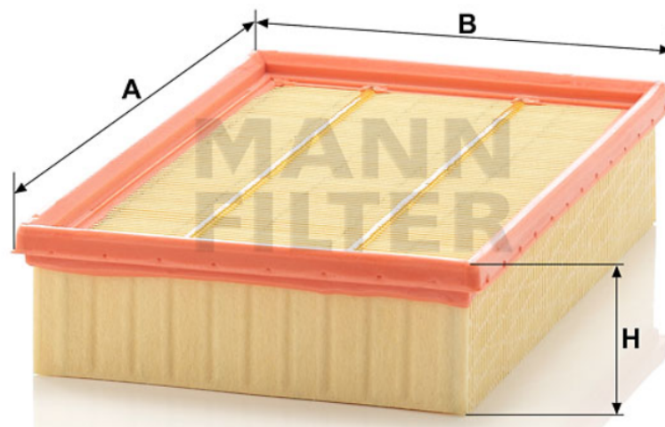
Filtr powietrza C28100
