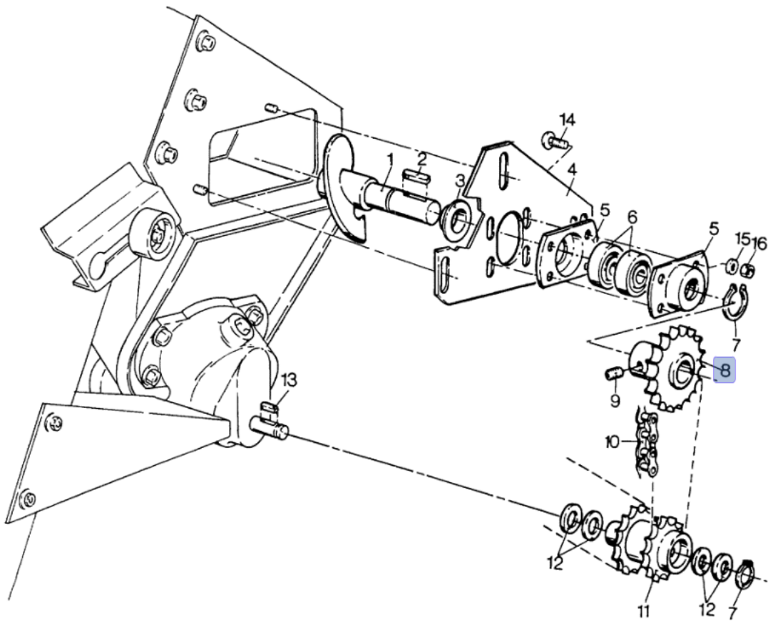
Koło łańcuchowe podajnik NH 423659
