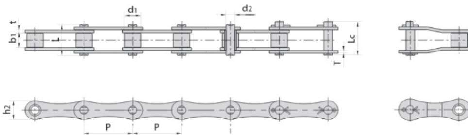
Łańcuch 208A 2040
