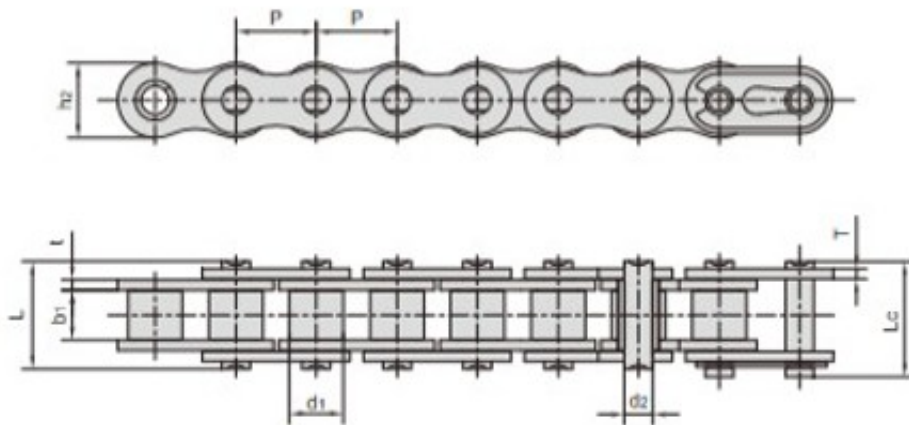
Łańcuch napędowy 420
