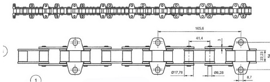
Łańcuch podajnik pochyły Claas WEW 38,4VB b8,3 fi-10
