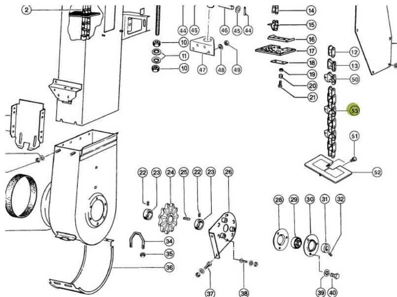
Łańcuch elewatora Class 795362.1
