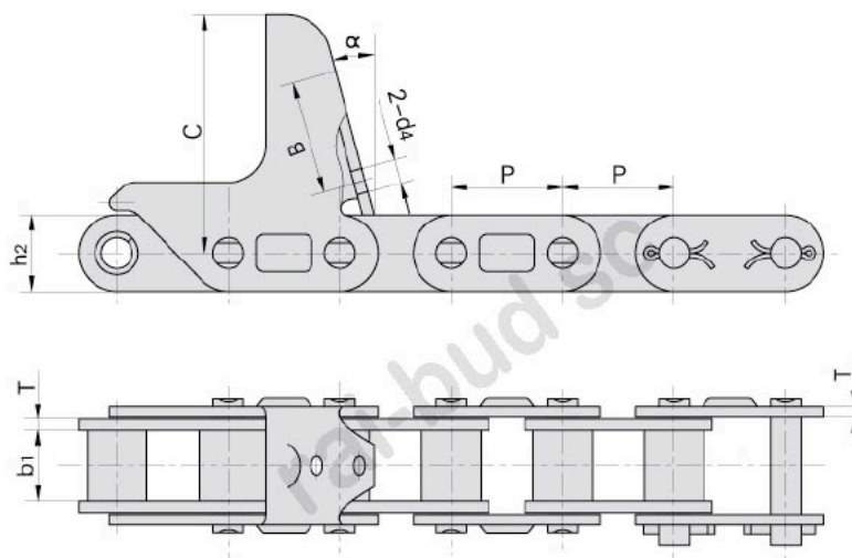
Łańcuch przystawka PC Gerringhoff 034850
