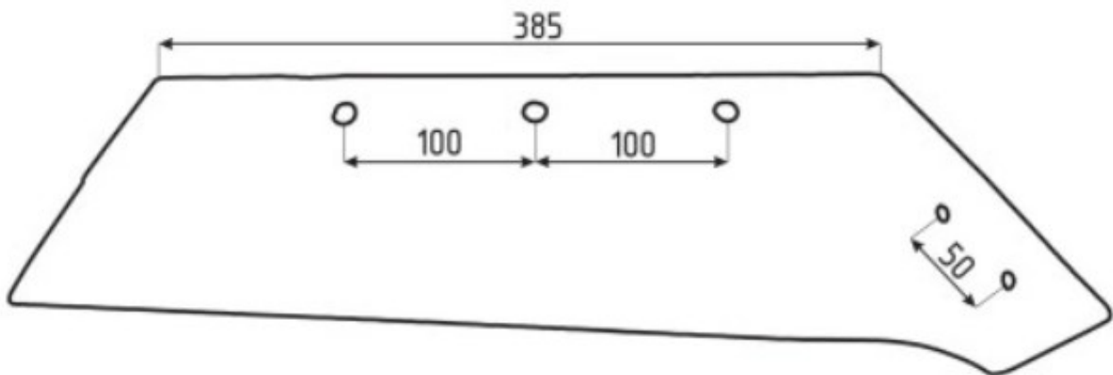
Lemiesz VN prawy WSM40 szerszy PREMIUM
